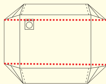
スタンディングテープ (赤い点線位置)
